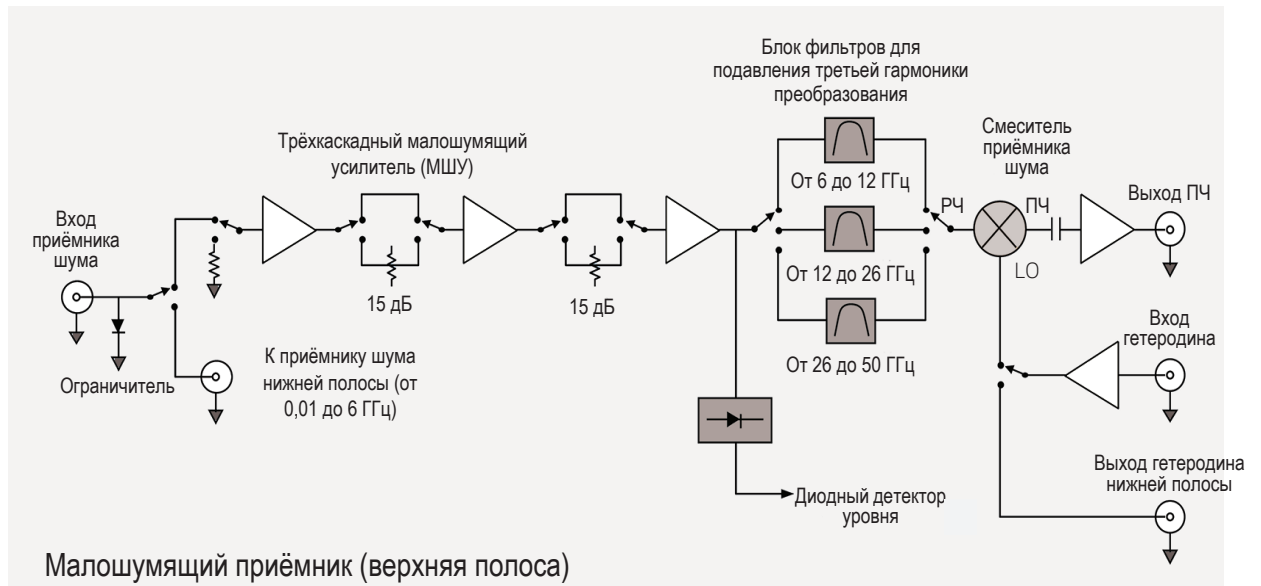
Рисунок 14 - В специализированном малошумящем приёмнике тракт сигнала, ведущий к смесителю, включает малошумящий усилитель блок фильтров.
