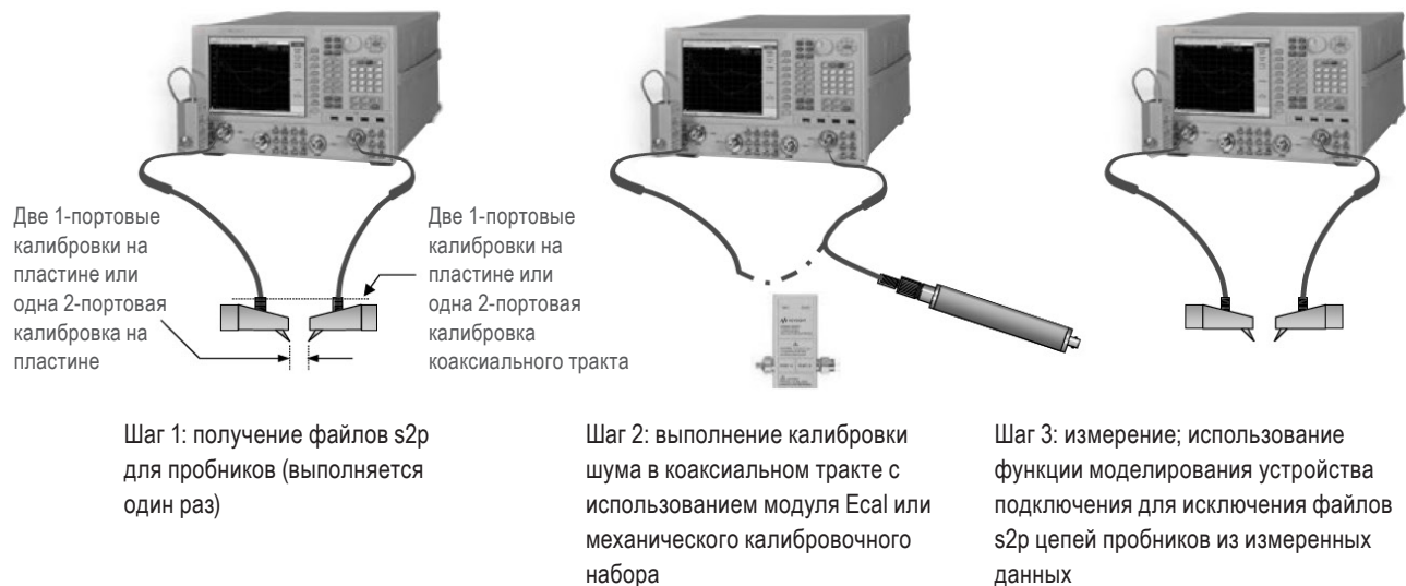
Рисунок 7 - Исключение цепей пробников зондовой станции представляет собой другой способ получения калиброванных результатов измерений.
