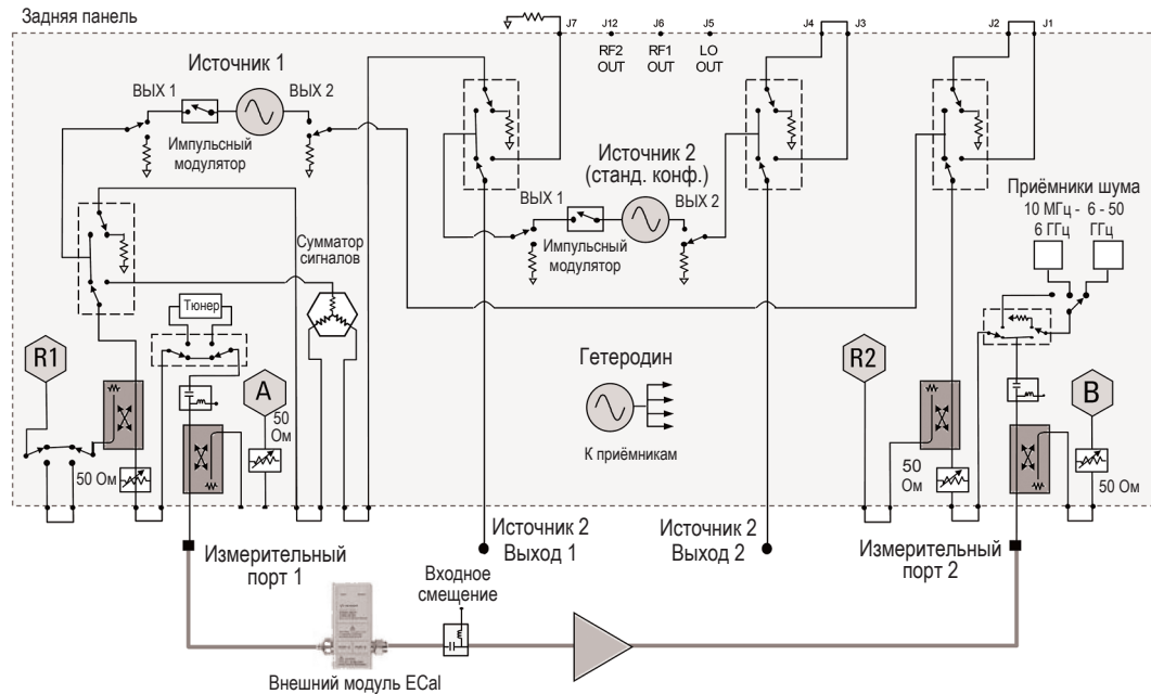
Рисунок 10 - Данная конфигурация с внешним тюнером и цепью подачи смещения помогает решить проблемы, связанные с потерями в кабелях, и позволяет провести более эффективную векторную калибровку шума. КОНТРОЛЯ.
