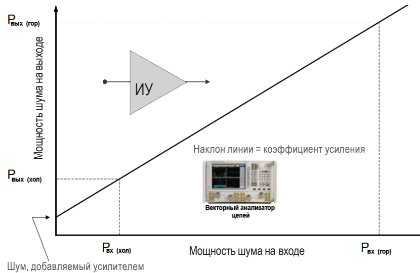
Рисунок 1 - График зависимости мощности шума на выходе от мощности шума на входе отображает информацию о коэффициенте усиления, линейности характеристики и внутреннем шуме усилителя.
