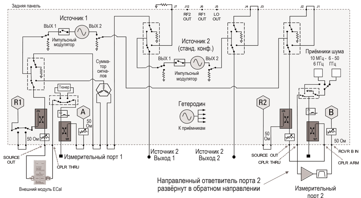
Рисунок 15 - Добавление внешнего предусилителя и фильтра улучшает качество измерений коэффициента шума с использованием стандартных приёмников в диапазоне частот от 50 до 67 ГГц.
