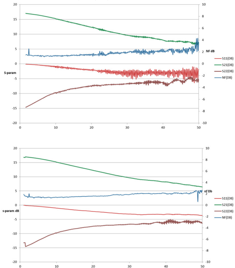
Рисунки 12a и 12b - По сравнению с результатами, приведёнными на рисунке 8b, данные графики, полученные на установке зондового контроля 1, показывают улучшения при измерении S-параметров и коэффициента шума.
