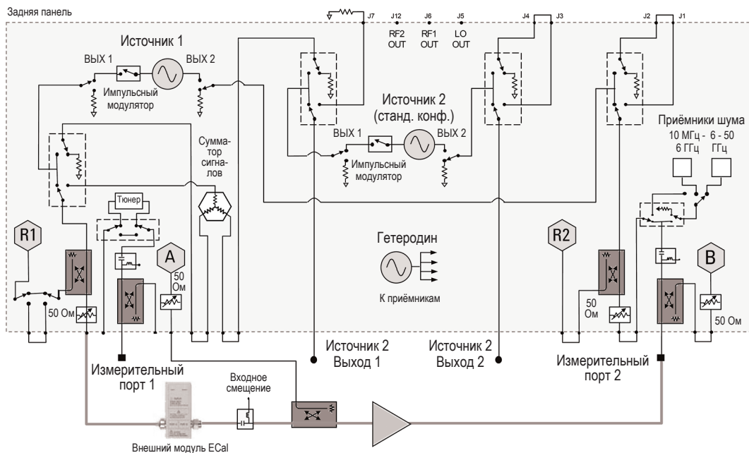
Рисунок 11 - В качестве меры по улучшению использования внешнего модуля ECal для оптимального расширения диапазона импедансов источника можно рассмотреть добавление внешнего направленного ответвителя и расположение его вблизи ИУ, что помогает сохранить нескорректированные характеристики направленности.
