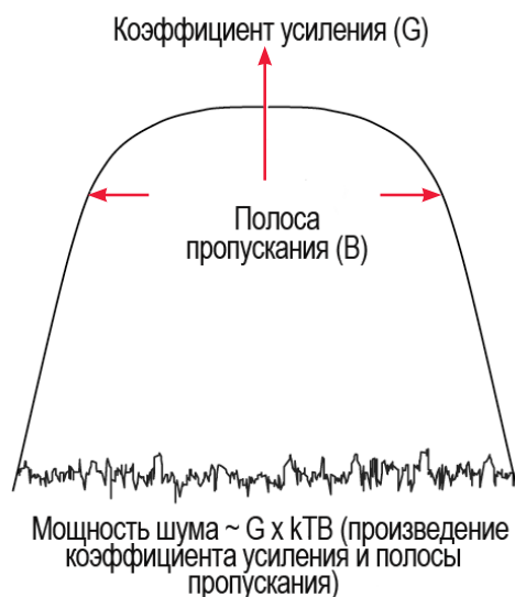
Рисунок 5. Определение произведения коэффициента усиления и полосы пропускания приёмника шума помогает измерить мощность шума, вносимую внутренними приёмниками шума, которая используется в качестве поправочного коэффициента для обеспечения калиброванных измерений.
