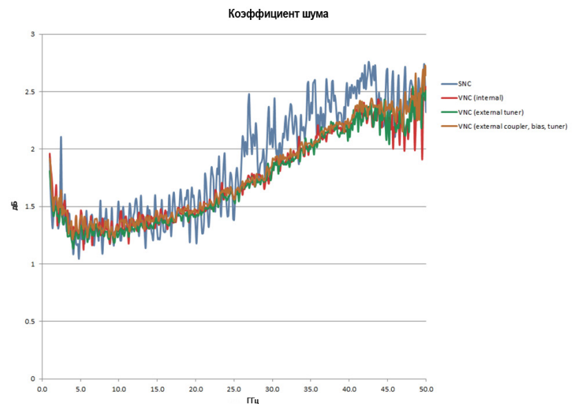
Рисунок 13 - Улучшения очевидны, но они не настолько существенны в случае с установкой зондового контроля 2 отчасти из-за качественных кабелей и хороших характеристик внутреннего тюнера.
