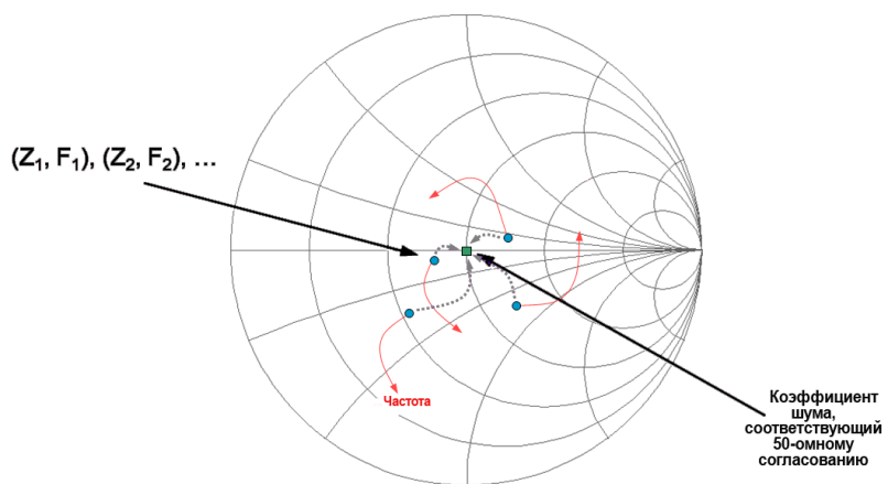
Рисунок 3 - Анализатор цепей серии PNA-X может использовать от четырёх до семи состояний импеданса, которые отличаются от 50 Ом, чтобы обеспечить точное вычисление коэффициента шума, соответствующего 50-омному согласованию в источнике, для ИУ.
