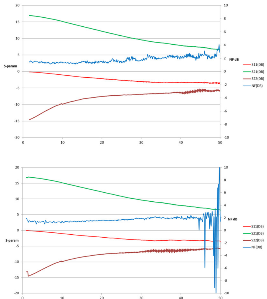
Рисунок 8a и 8b - В сравнении со скалярной калибровкой шума (вверху) векторная калибровка шума снижает неравномерность характеристики, имеющей вид пульсаций, при измерениях коэффициента шума (NF) (графики синего цвета).
