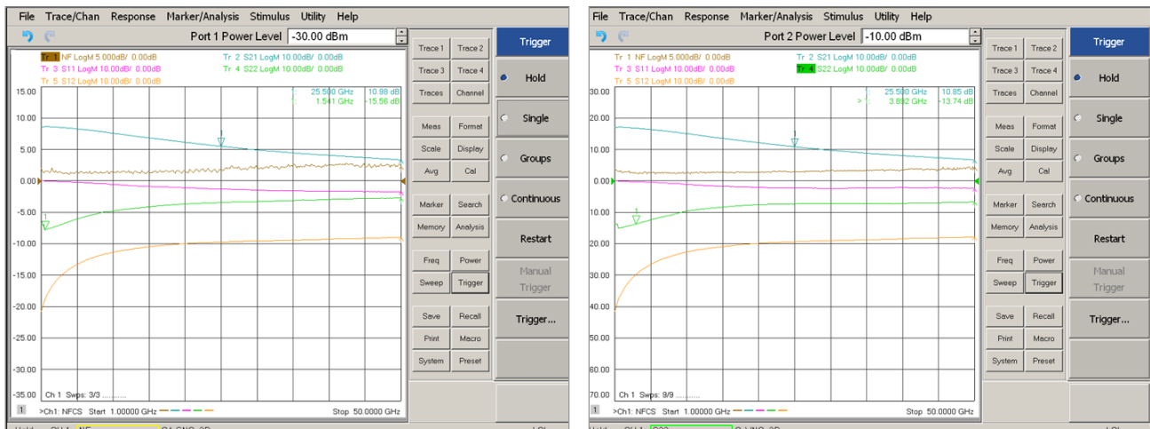
Рисунок 9 - Использование высококачественных кабелей и векторного анализатора цепей с лучшим коэффициентом шума позволяет получить точные, без пульсаций, результаты измерений с помощью векторной калибровки шума (графики, расположенные справа).
