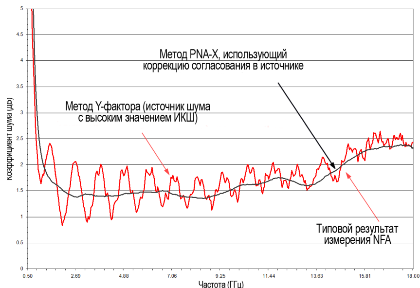
Рисунок 4 - Используя метод коррекции согласования в источнике, анализатор цепей серии PNA-X обеспечивает более точное представление коэффициента шума ИУ по сравнению с использованием типового метод Y-фактора и анализатора коэффициента шума серии NFA.
